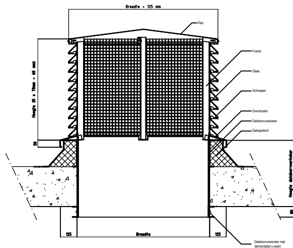
Doorsnede
