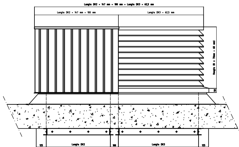
Zijaanzicht
