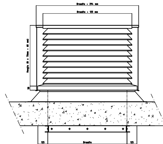
Zijaanzicht
