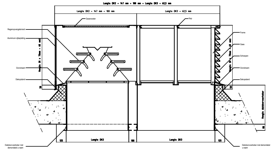
Doorsnede
