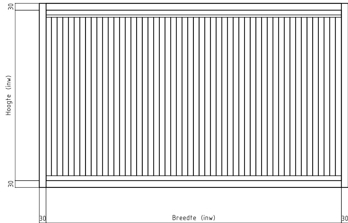
Vooraanzicht
