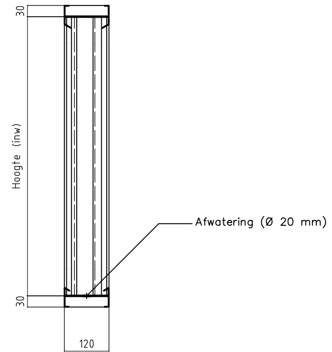
Doorsnede
