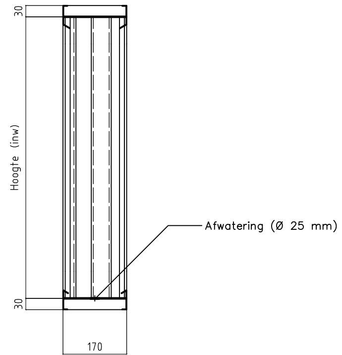
Doorsnede
