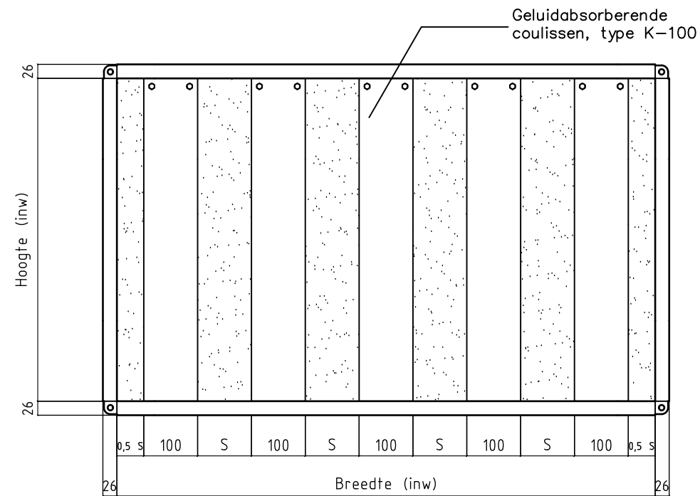
Vooraanzicht
