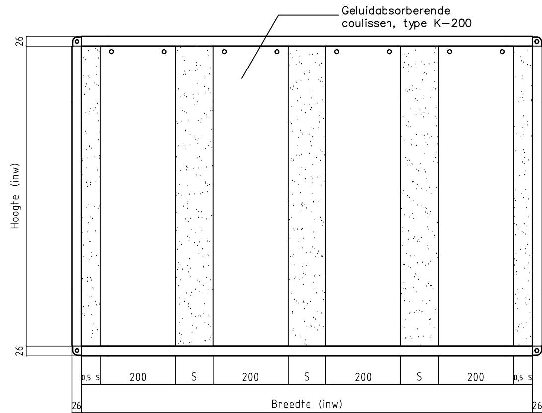
Vooraanzicht
