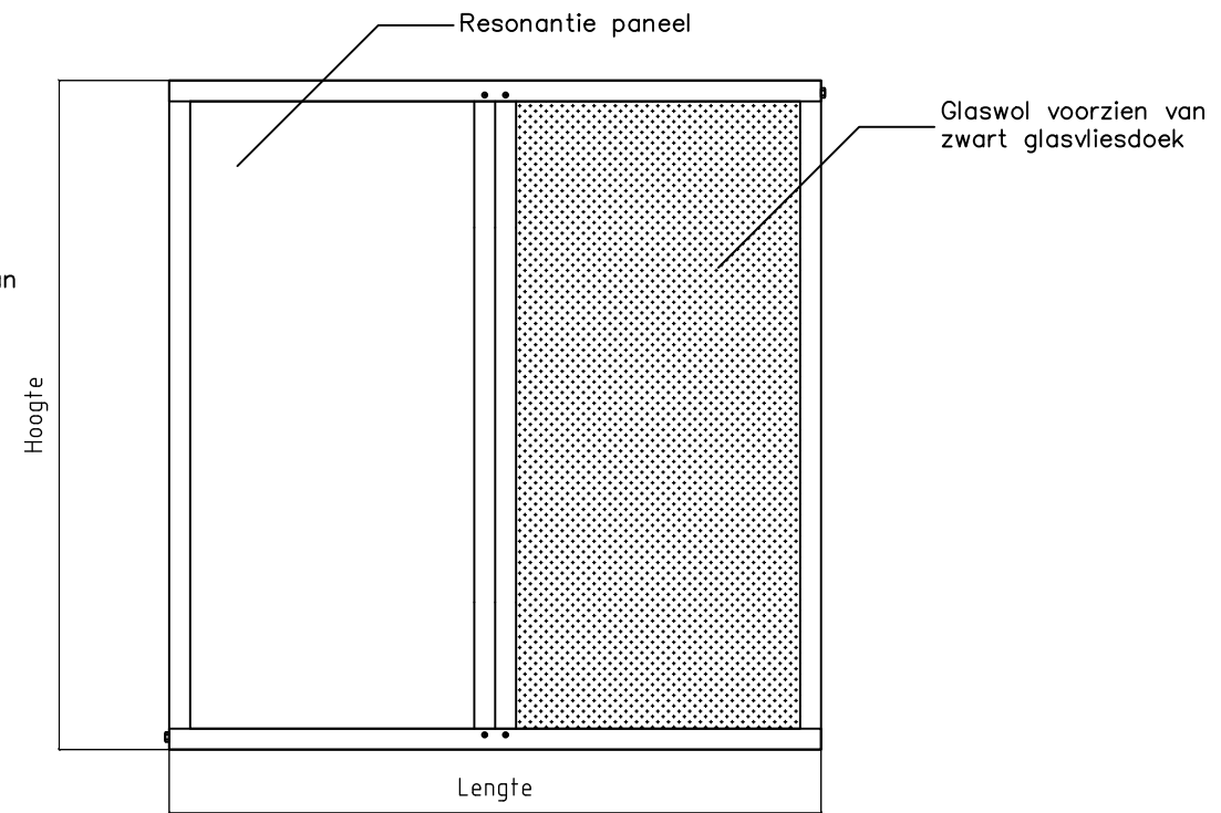
Zijaanzicht
