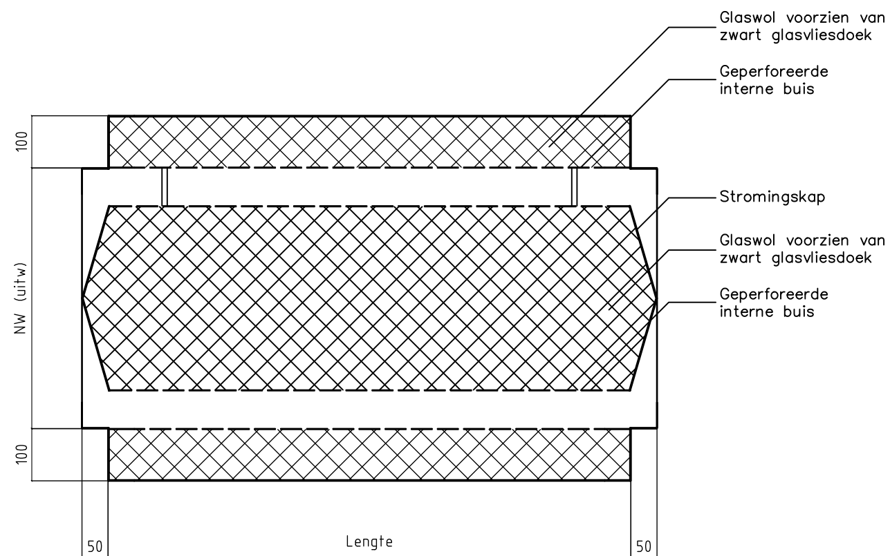
Doorsnede
