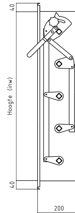
Zijaanzicht
