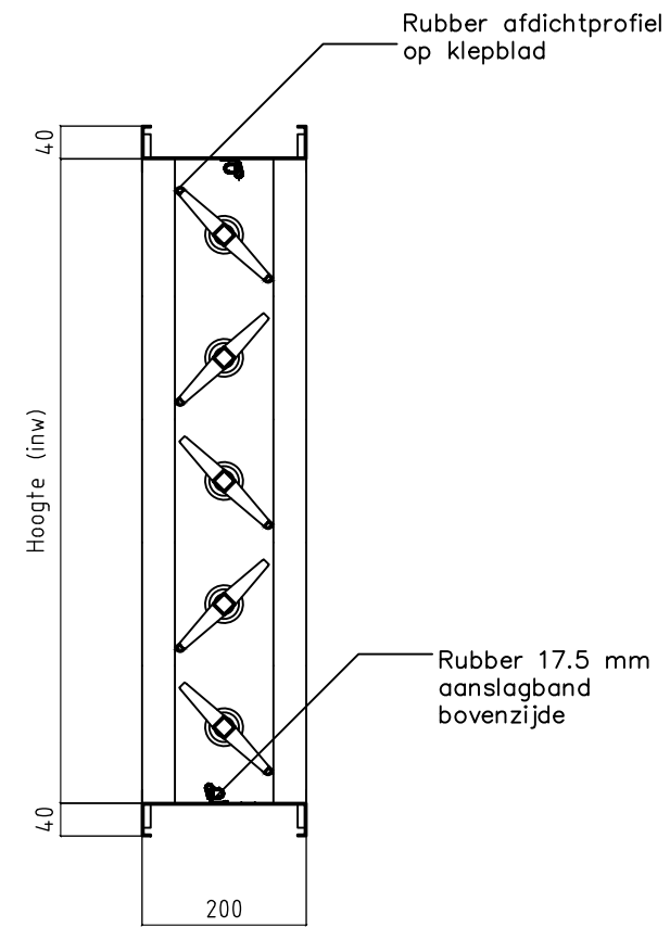
Doorsnede
