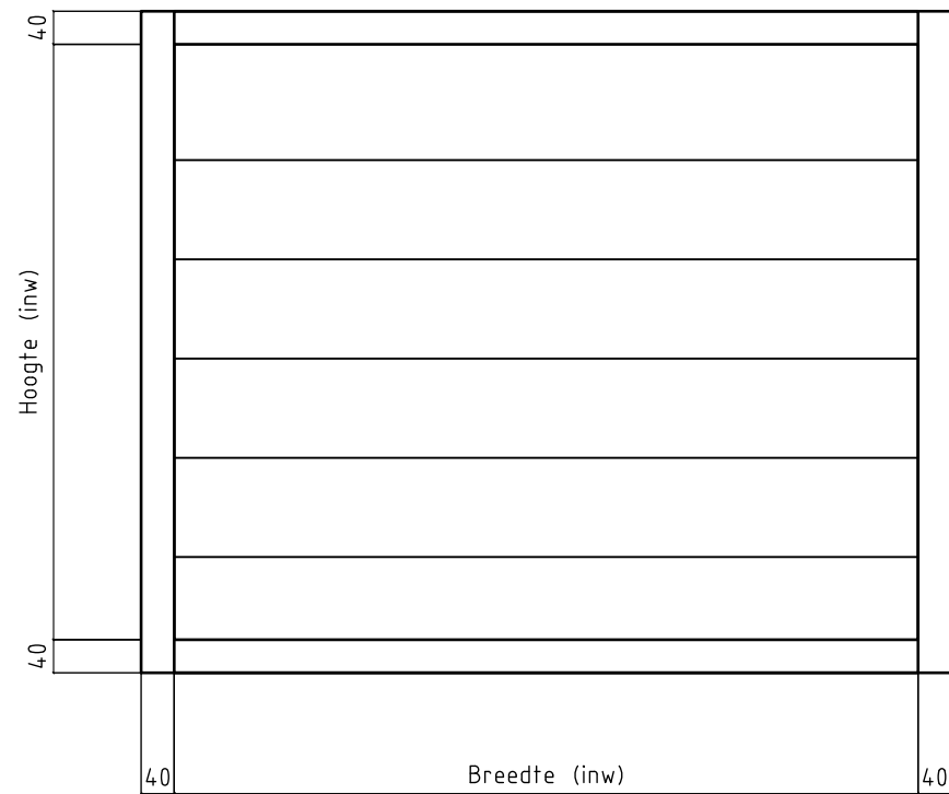
Vooraanzicht
