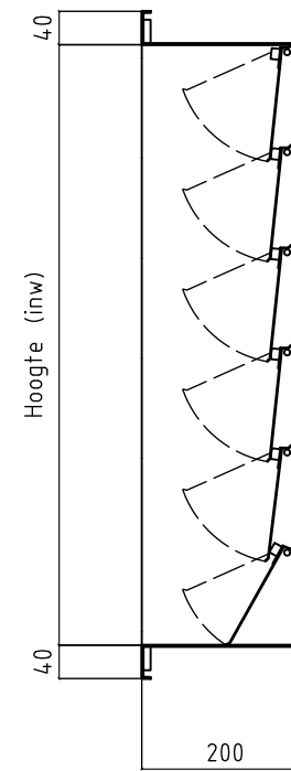
Doorsnede
