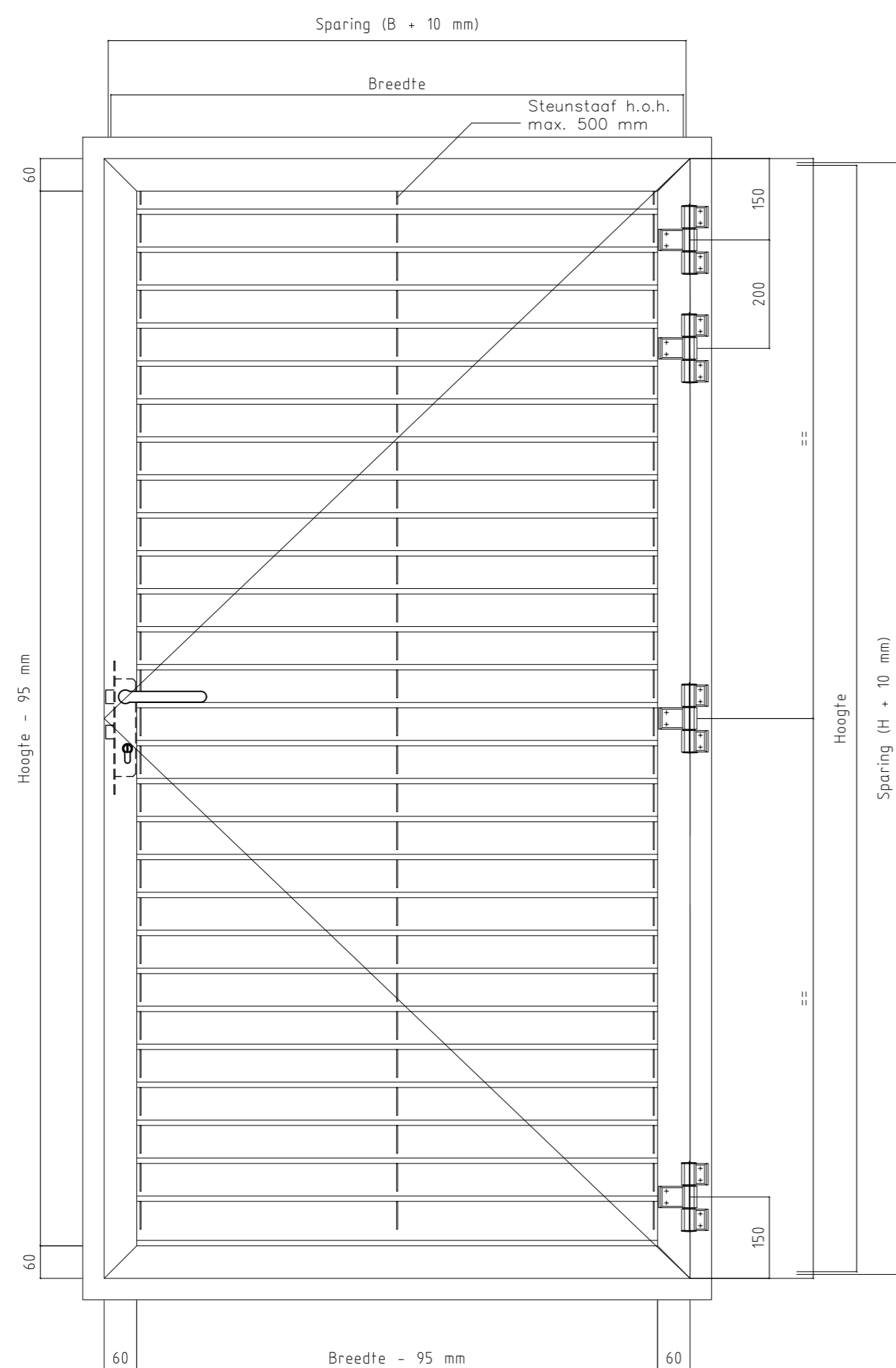
Vooraanzicht
